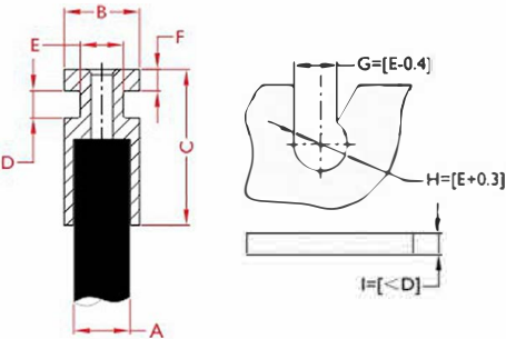
推荐配合槽尺寸 Recommended groove size
